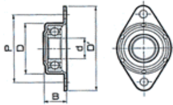
菱フランジユニット
